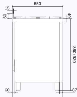
Vista laterale P36N / P36W
